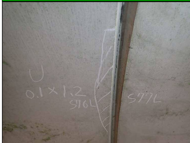
【施 工 後(補修状況)】
