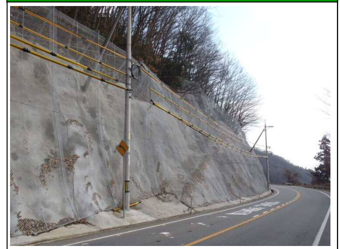
【施 工 後】
