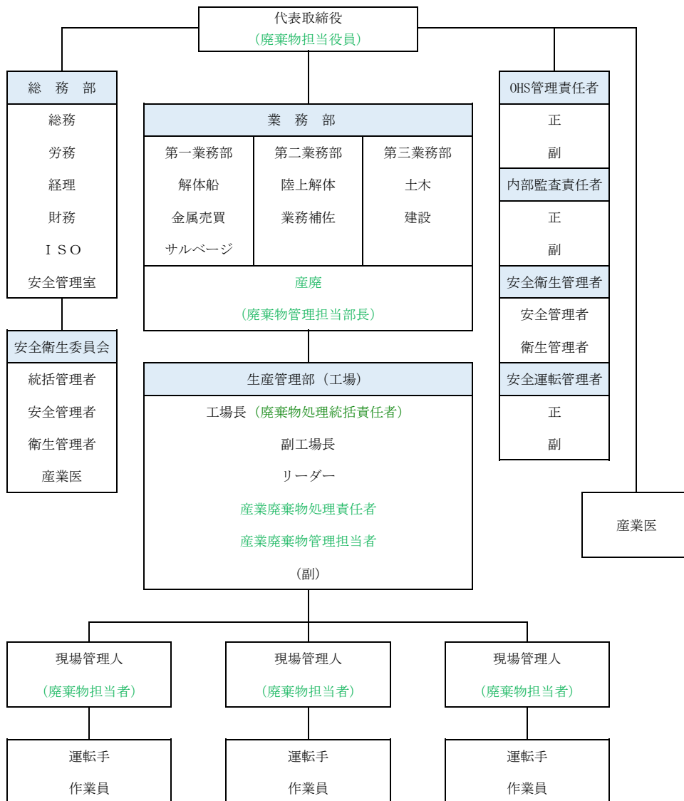
管理体制図
