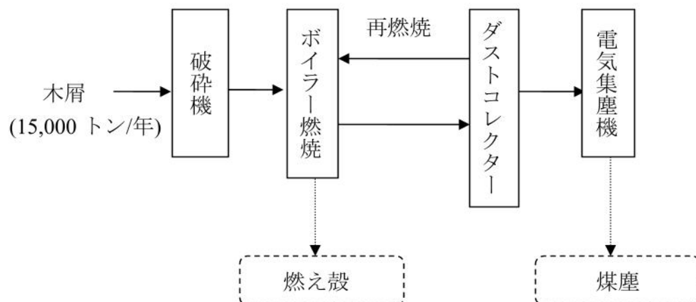
図 2 ドライクリーニング廃液、汚泥発生フローシート
