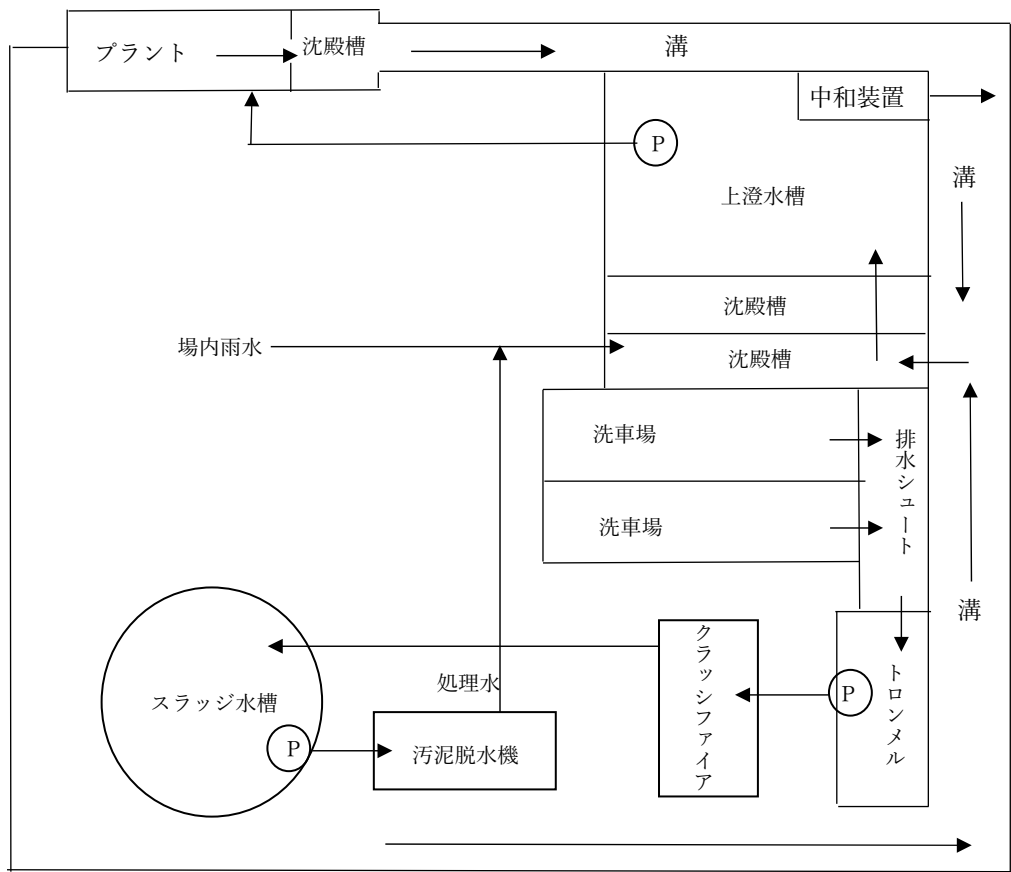
図 1 排水処理フローシート
