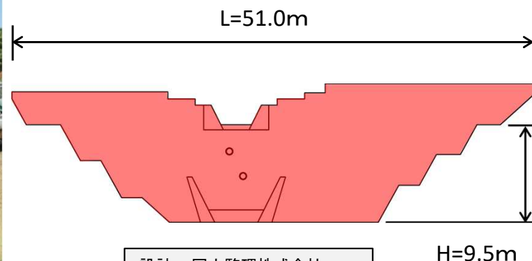
堰堤一般図
