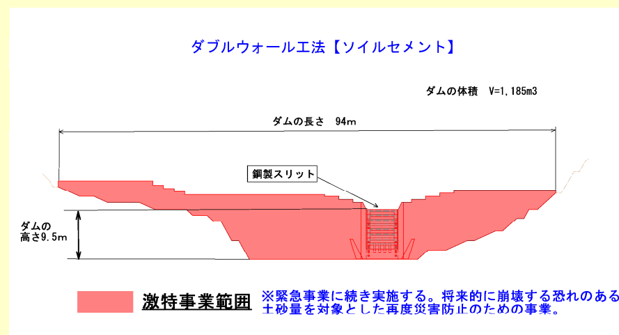
【正面図】
