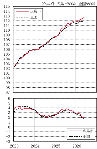
図4 生鮮食品及びエネルギーを除く総合指数、前年同月比の推移 2023.1～2026.5
