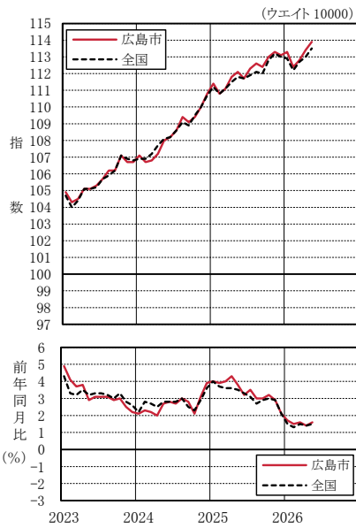
図2 総合指数、前年同月比の推移 2023.1～2026.5
