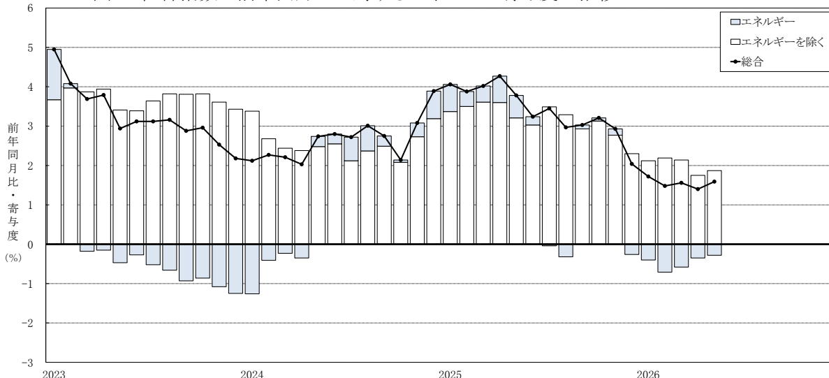
図6 総合指数の前年同月比に対するエネルギー寄与度の推移 2023.1~2026.5
