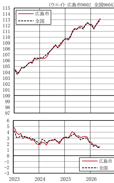
図3 生鮮食品を除く総合指数、前年同月比の推移 2023.1～2026.5
