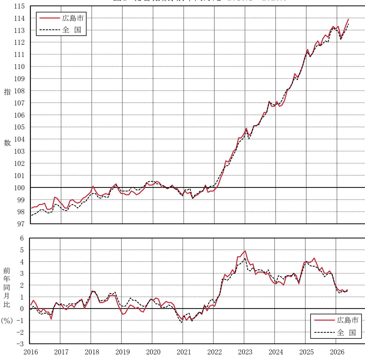
図1 総合指数、前年同月比 2016.1~2026.5
